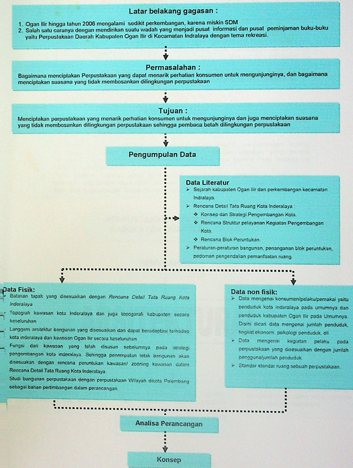
Gambar 1 Kerangka Berpikir
