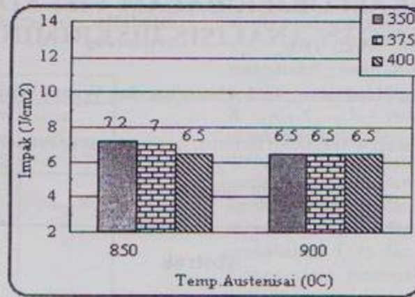
Gambar 14. Impak Vs. temp. austenisasi untuk sampel B
