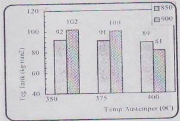
Gambar 9. Teg. tarik Vs. temp. austemper untuk sampel A
