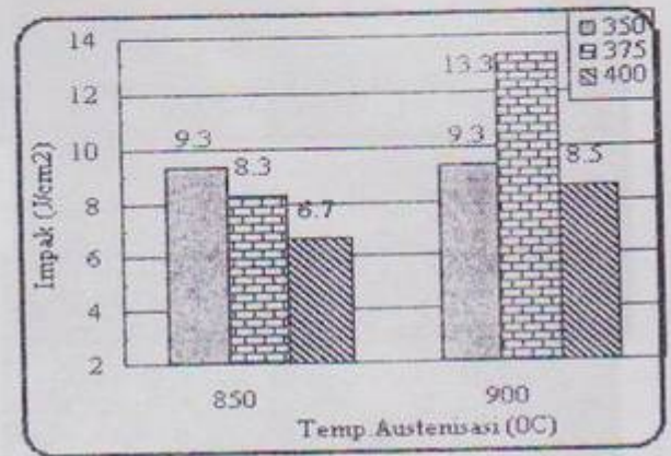
Gambar 13. Impak Vs. temp. austemisasi untuk sampel A
