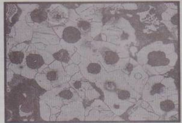
Gambar 2. Foto struktur as-cast B pembesaran 200 X
