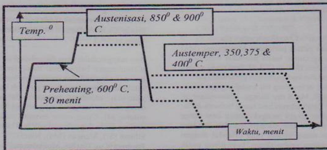
Gambar 1. Skematis proses perlakuan panas
