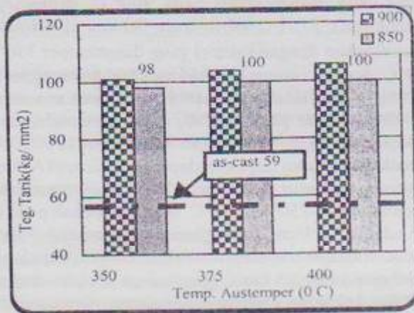
Gambar 10. Teg. tarik Vs. temp. austemper untuk sampel B
