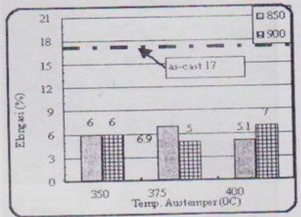
Gambar 11. Elongasi Vs. temp. austemper untuk sampel A
