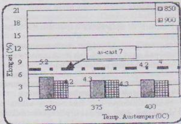
Gambar 12. Elongasi Vs. temp. austemper untuk sampel B
