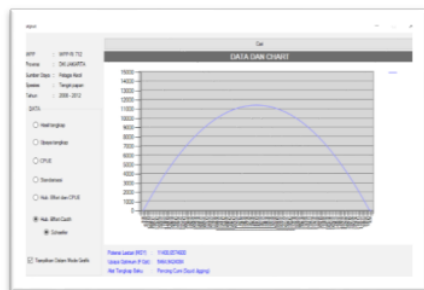
Gambar 11. Sub program Output/Proses MSY, Fmsy, Alat tangkap baku dan Grafik hubungan upaya tangkap terhadap hasil tangkap menggunakan model schaefer
