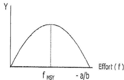
Gambar 1. Grafik Hubungan Hasil Tangkap dan Upaya Tangkap
