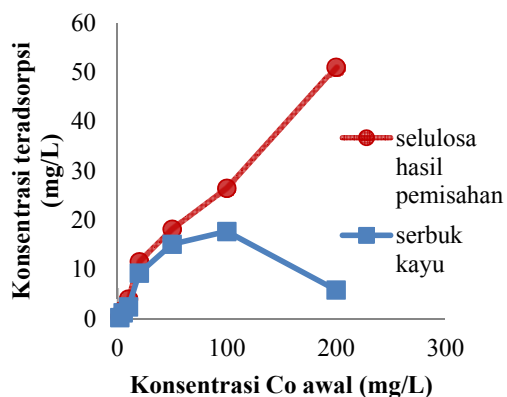
Gambar 3. Pengaruh konsentrasi pada interaksi ion logam \text{Co}^{2+} dengan selulosa hasil ekstraksi dan serbuk gergaji kayu.
