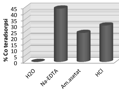
Gambar 4. Desorpsi ion logam \text{Co}^{2+} pada adsorben selulosa
