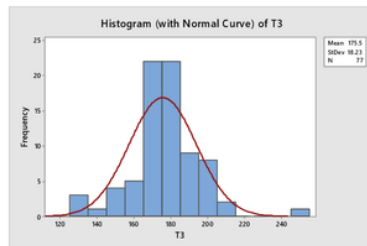
(d) Histogram T3
