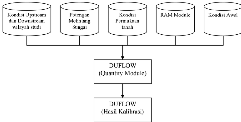
Gambar 3.3. Diagram Input-Output dalam pemodelan DUFLOW
