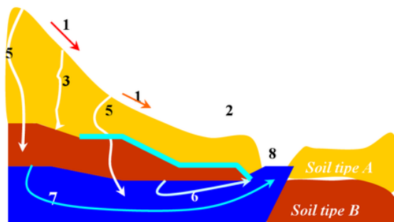
Gambar 2.2. Skema proses runoff pada daerah berlereng pada suatu DAS Sumber : Rientjes (2007)
