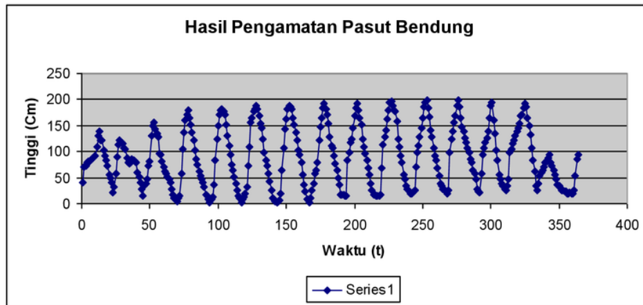
Gambar 5.6. Hasil Pengamatan Pasang Surut Sungai Bendung
