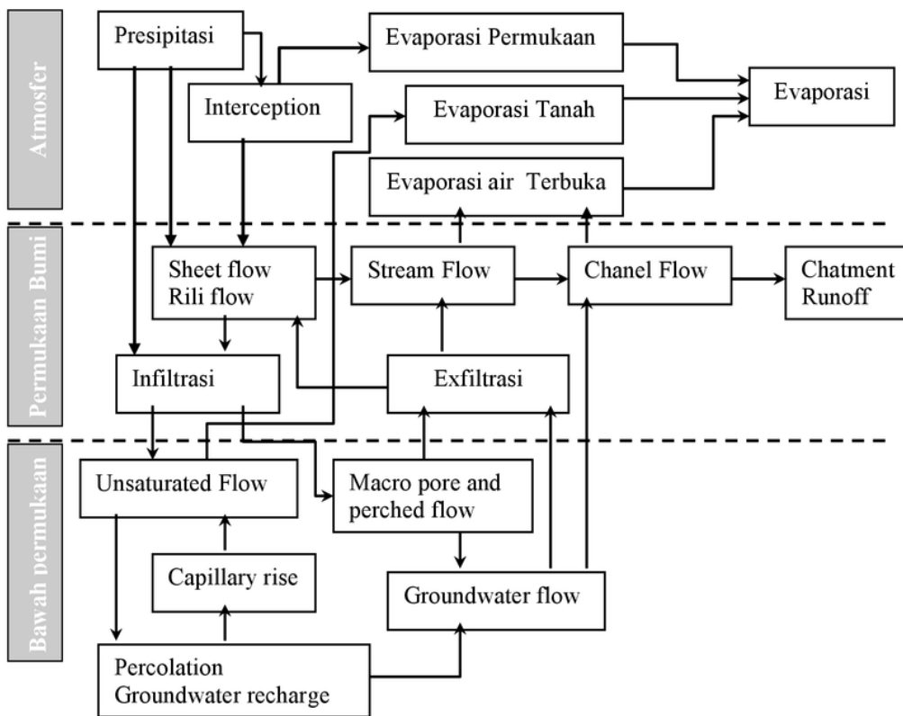
Gambar 2.1. Proses Utama secara diagramatik Siklus Hidrologi pada sistem DAS
