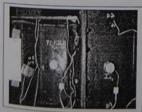
(a) Flush End-Plate
