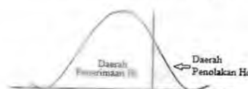
Gambar 1. Daerah Penerimaan dan Penolakan Hipotesis
