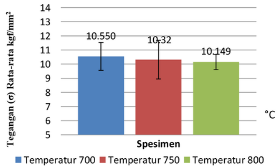
Gambar 6. Tegangan Vs Temperatur Penuangan
