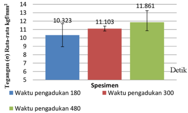
Gambar 5. Tegangan VS waktu pengadukan
