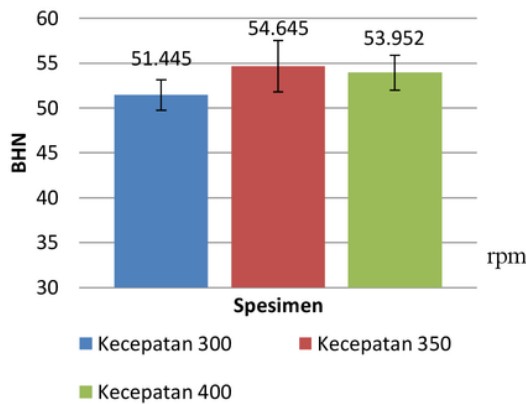
Gambar 11. Kekerasan rata-rata VS Kecepatan stir
