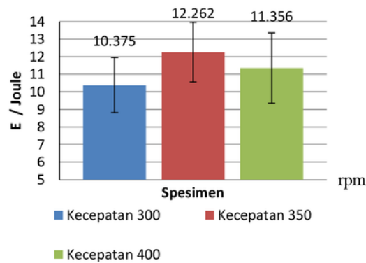
Gambar 3. Grafik; E rata-rata VS Kecepatan Stir
