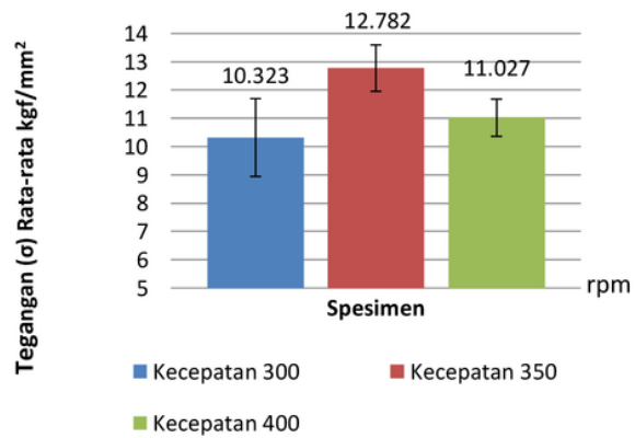
Gambar 7. Tegangan VS Kecepatan stir
