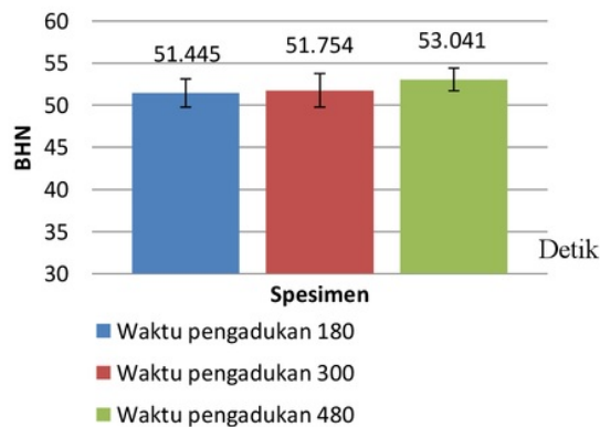
Gambar 9. Kekerasan VS waktu pengadukan
