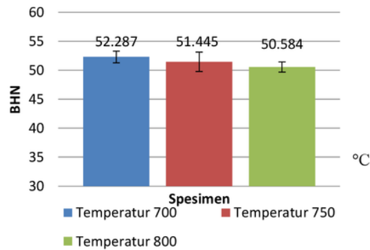
Gambar 10. Kekerasan rata-rata VS Temperatur Penuangan
