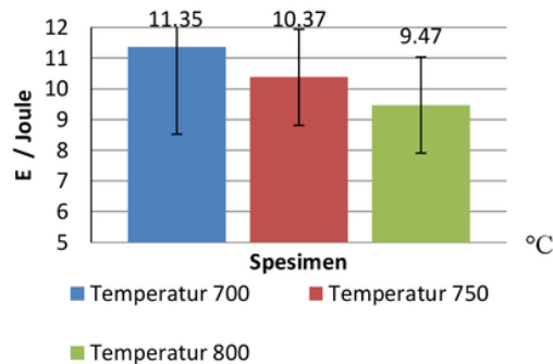
Gambar 2. Grafik; E VS Temperatur Penuangan
