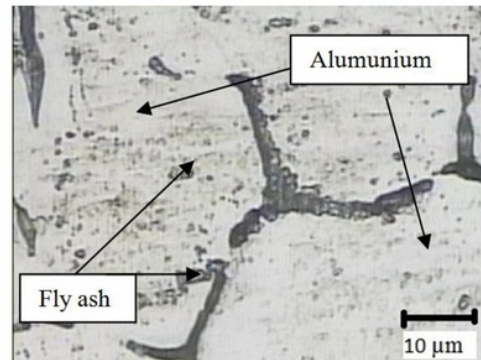
Gambar 12 Hasil struktur mikro dengan komposisi Alumina 8% dan fly ash 12%
