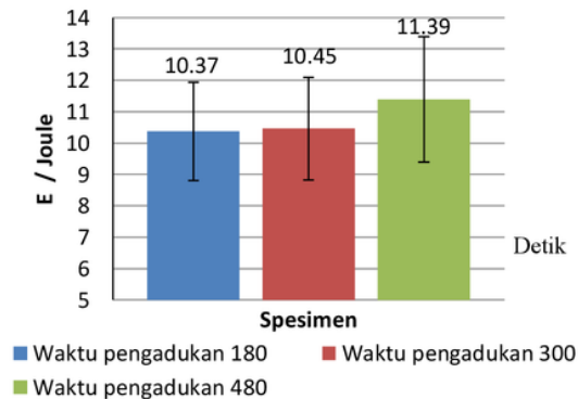
Gambar 1. Grafik; E rata-rata VS Waktu pengadukan (detik)
