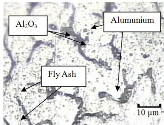
Gambar 13 Hasil struktur mikro pembesaran
