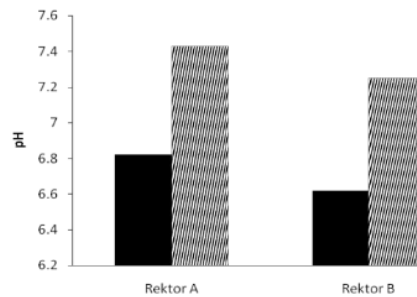
Gambar 1. Nilai pH Slurry .
