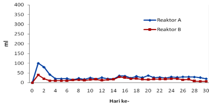
Gambar 10. Grafik pembentukan metana per hari.
