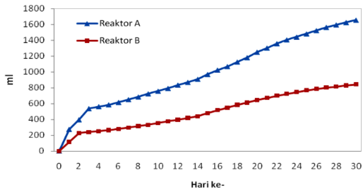
Gambar 8. Grafik akumulasi volume produksi biogas.
