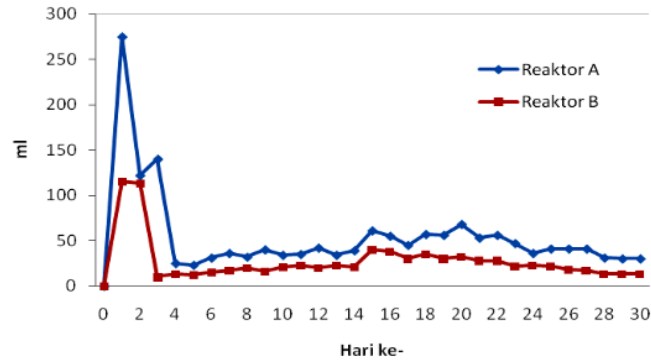
Gambar 11. Grafik pembentukan biogas per hari.
