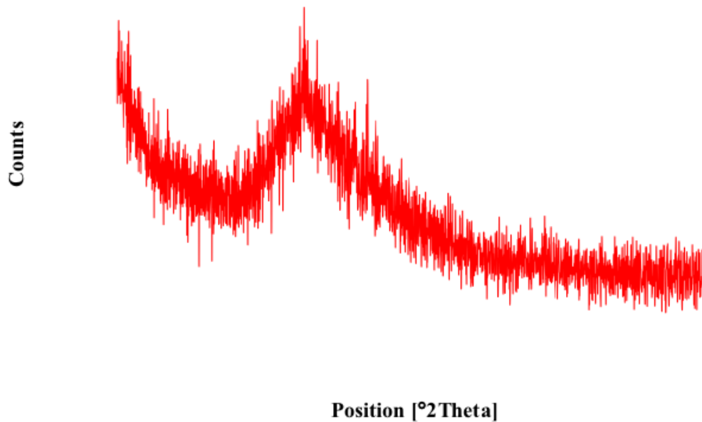
Fig. 2. XRD bagasse ash.
