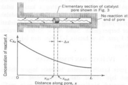
Gambar 4. Profil penurunan konsentrasi reaktan sepanjang volume katalis.
