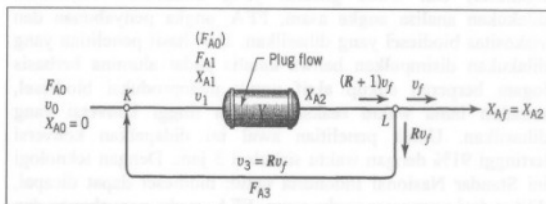
Gambar. 1 Nomenklatur Recycle Reactor (Leven Spiel)
