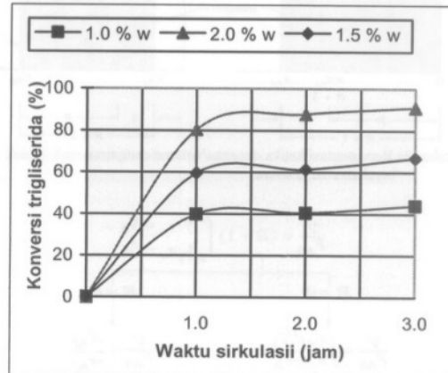
Gambar.5. Pengaruh % berat katalis padat terhadap konversi trigliserida menjadi biodiesel didalam fixed bed reaktor recycle
