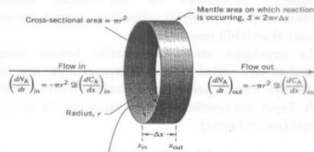
Gambar 3. Tahapan proses reaksi katalitik perelemen pori katalis
