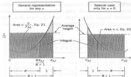
Gambar 2a. Representasi ketika densitas/volume campuran reaksi tidak berubah atau konstan
