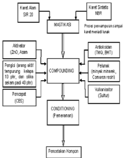
Gambar 1. Tahapan Proses Pembuatan kompon karet
