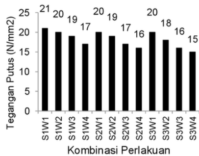
Gambar 4. Tegangan Putus (N/mm 2 ) Kompon Karet Setelah Pengusangan
