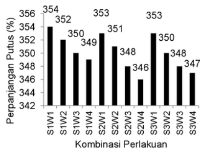
Gambar 5. Perpanjangan Putus (N/mm 2 ) Kompon Karet Setelah Pengusangan
