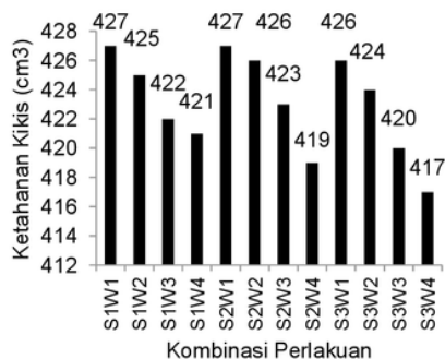
Gambar 6. Ketahanan Kikis (cm 3 ) Kompon Karet Setelah Pengusangan
