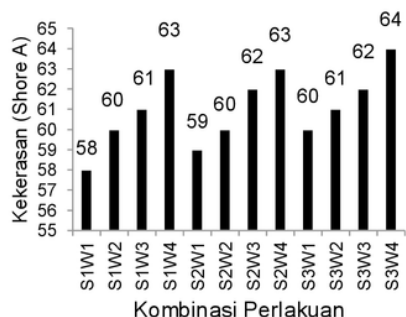
Gambar 2. Kekerasan(ShoreA) Kompon Karet Setelah Pengusangan
