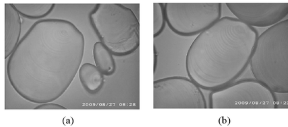
Gambar 1. Bentuk granula pati ganyong dengan perbesaran 1000x a) sebelum modifikasi dan b) setelah modifikasi 0,12% \text{POCl}_3
