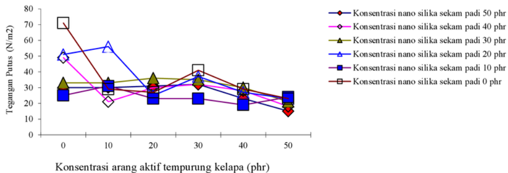
Gambar 2. Tegangan putus ( N/mm^2 ) kompon karet
