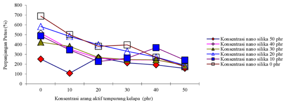
Gambar 4. Perpanjangan putus (%) kompon karet
