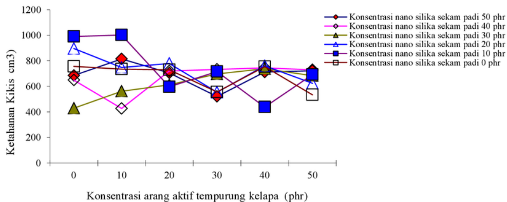
Gambar 5. Ketahanan kikis ( cm^3 ) kompon karet
