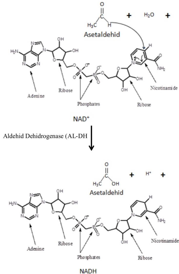
Gambar 2. Reaksi oksidasi asetaldehid (Boeringer Mannheim, 2011)
