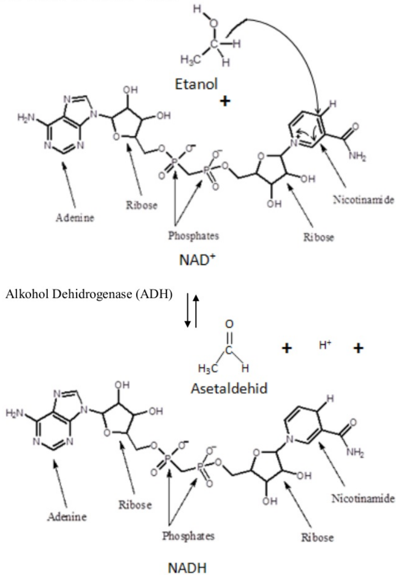
Gambar 1: Reaksi oksidasi etanol (Boeringer Mannheim, 2011)
