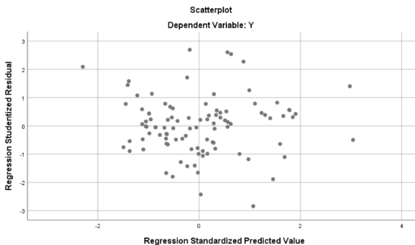
Gambar 4.4 Uji Heteroskedastisitas Model Regresi II
