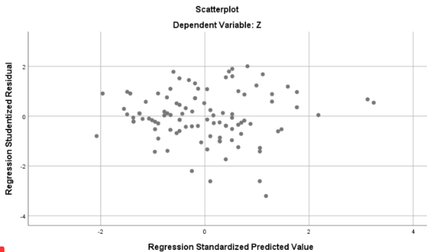
Gambar 4.3 Uji Heteroskedastisitas Model Regresi I
