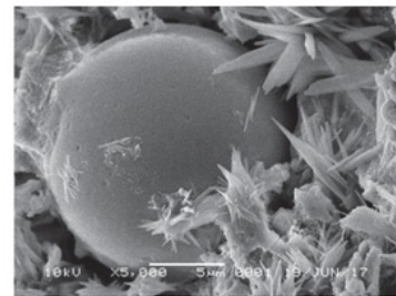
(d) \text{Na}_2\text{SiO}_3/\text{NaOH} 3.25
