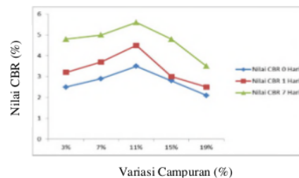
Gambar 4. Grafik Nilai CBR US Tanah Campuran
