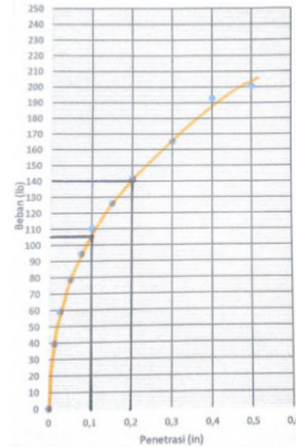
Gambar 3. Grafik CBR US Tanah Asli
