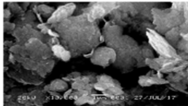
Gambar 5. Hasil Pengujian SEM Tanah Asli
