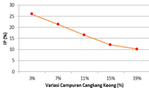
Gambar 2. Grafik Nilai IP Tanah Campuran
