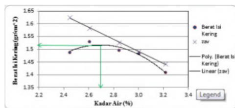
Gambar 1. Grafik Pemadatan Standar Tanah Asli (Yesumpo, 2017)
