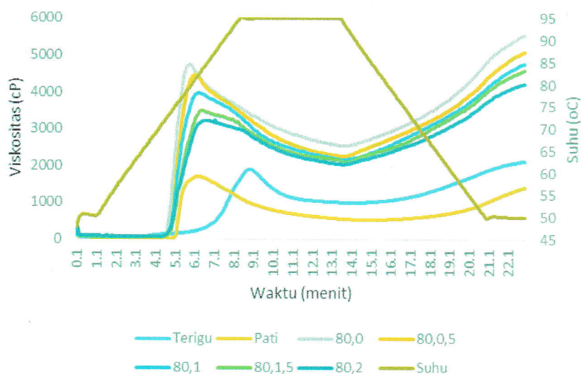
Gambar 1. Viskositas pati ganyong termomodifikasi pada suhu HMT 80°C.
