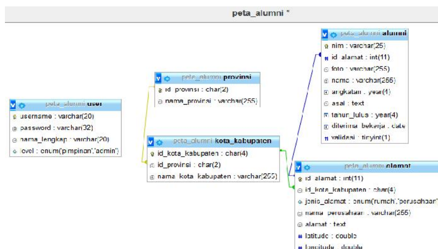
Gambar 5.9 Skema Database
