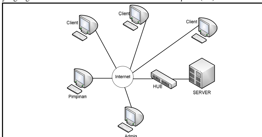
Gambar 5.8 Arsitektur Sistem
