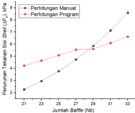
Gambar 2 Penurunan Tekanan Sisi Shell
