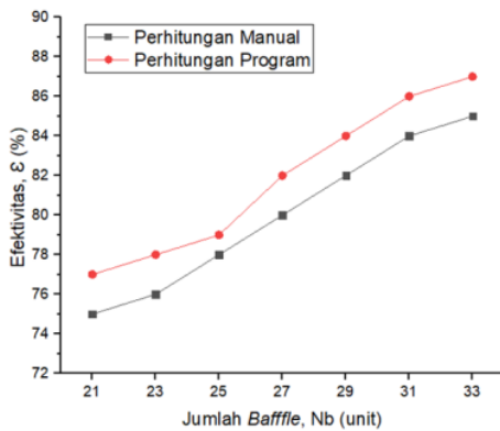
Gambar 11 Efektivitas Penukar Kalor dan Jumlah Baffle
