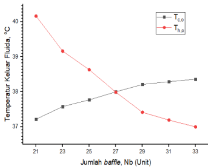
Gambar 10 Temperatur Keluar Fluida dan Jumlah Baffle
