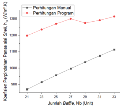
Gambar 5 Koefisien Perpindahan Panas Shell
