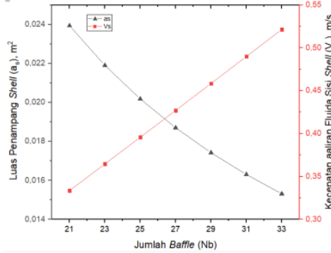
Gambar 7 Luas Penampang dan Kecepatan Aliran Fluida shell
