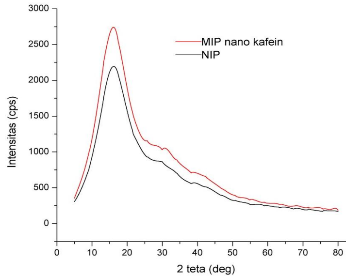
Gambar 2. Pola XRD dari NIP dan MIP
