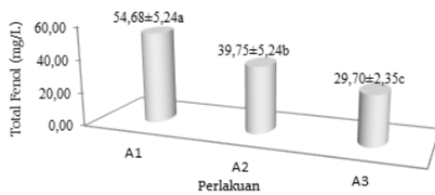
Gambar 5. Nilai rerata kadar total fenol (mg/L) daun tanaman gaharu; A1= daun muda (posisi daun 1-4 helai dari pucuk); A2= daun sedang (posisi daun 5-8 helai dari pucuk); A3= daun tua (posisi daun 9-11 helai dari pucuk); angka-angka yang diikuti huruf kecil yang berbeda pada Gambar menunjukkan berbeda nyata.
