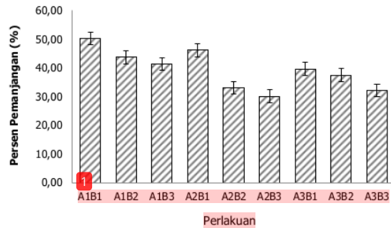
Gambar 2. Persen pemanjangan bioactive edible film
