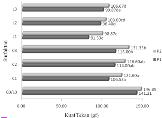
2 Gambar 2. Nilai rata-rata laju transmisi uap air edible film pati ganyong sebelum dan setelah CMC dan lesitin (P = pati g 11 ng, P 1 = sebelum modifikasi, P 2 = setelah modifikasi 13 = CMC, C 1 = 1 %, C 2 = 2 %, dan C 3 = 3 % (b/v). L = lesitin, L 1 = 0,20 %, L 2 = 0,25 %, dan L 3 = 0,30 %, dan C0/L0 = tanpa surfaktan)
