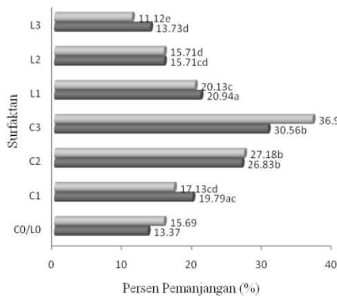
Gambar 3. Nilai rata-rata persen pemanjangan edible film setelah dan sebelum penambahan lilin lebah, CMC, dan lesitin (P1=pati sebelum modifikasi, P2=pati setelah modifikasi, C1, C2, dan C3 = konsentrasi CMC masing-masing 1 %, 2 %, dan 3 %, L1,L2, dan L3 = konsentrasi lesitin masing- masing 0,20 %, 0,25 %, dan 0,30 %, CO/L0 = tanpa surfaktan dan lilin lebah).
