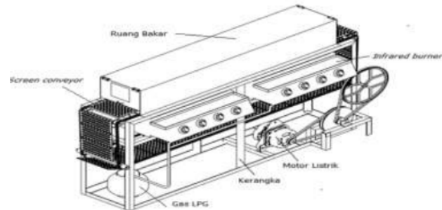
Gambar 3. Mesin pemanggang kemplang
