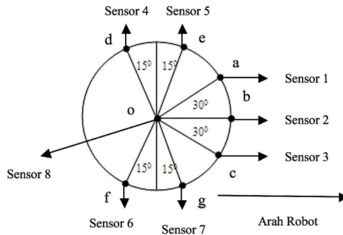
Gambar 4.4. Model Robot Berdasarkan Posisi Sensor
