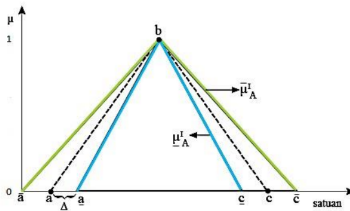
Gambar 5.8. Parameter-Parameter Pada Fungsi Keanggotaan Segitiga
