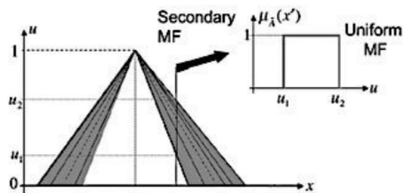
Gambar 3.7 Himpunan Fuzzy Interval Tipe-2 (Karnik & Mendel, 2009)
