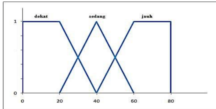
Gambar 5.1. Fungsi Keanggotaan Jarak
