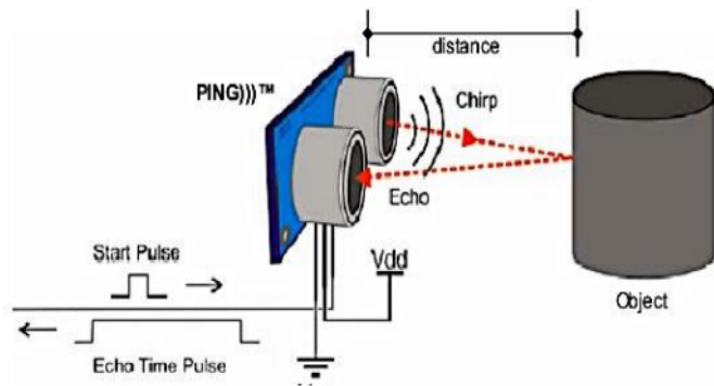
Gambar 2.1. Ilustrasi Cara Kerja Sensor Ultrasonik
