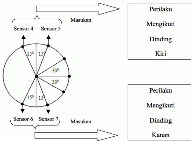
Gambar 4.13. Model Prilaku Mengikuti Dinding
