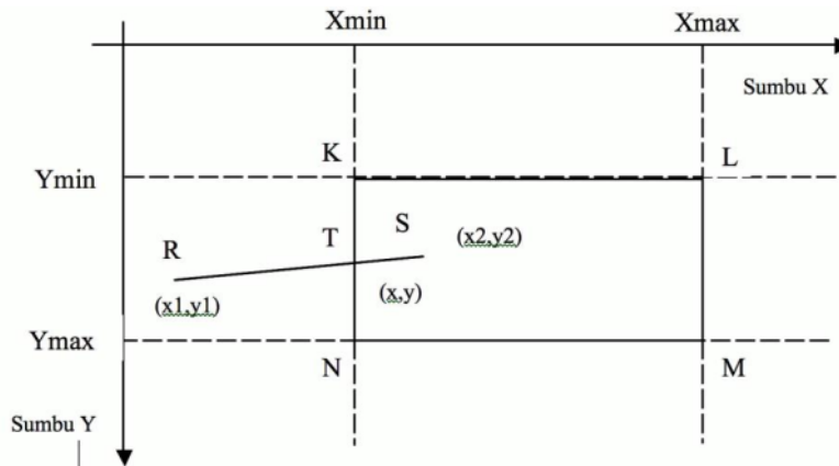
Gambar 4.8 Pemodelan Algoritma Liang-Barsky
