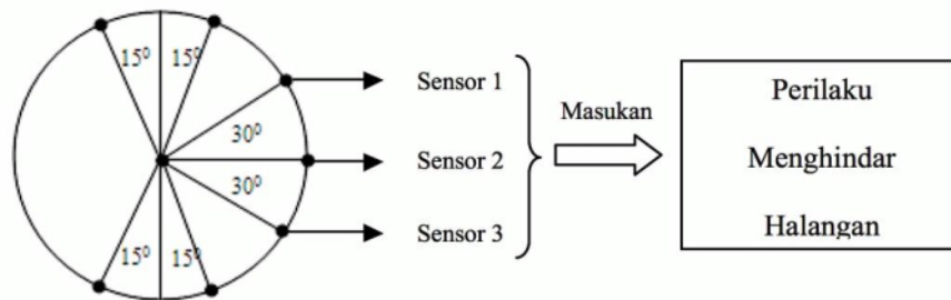
Gambar 4.11. Model Prilaku Menghindar Halangan
