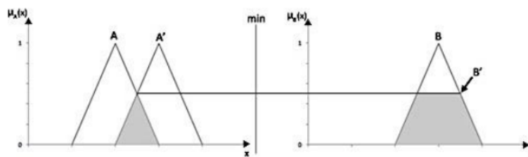
Gambar 3.2 Penalaran GMP pada kaidah tunggal dan antecedent tunggal (Castilo dan Melin, 2008)
