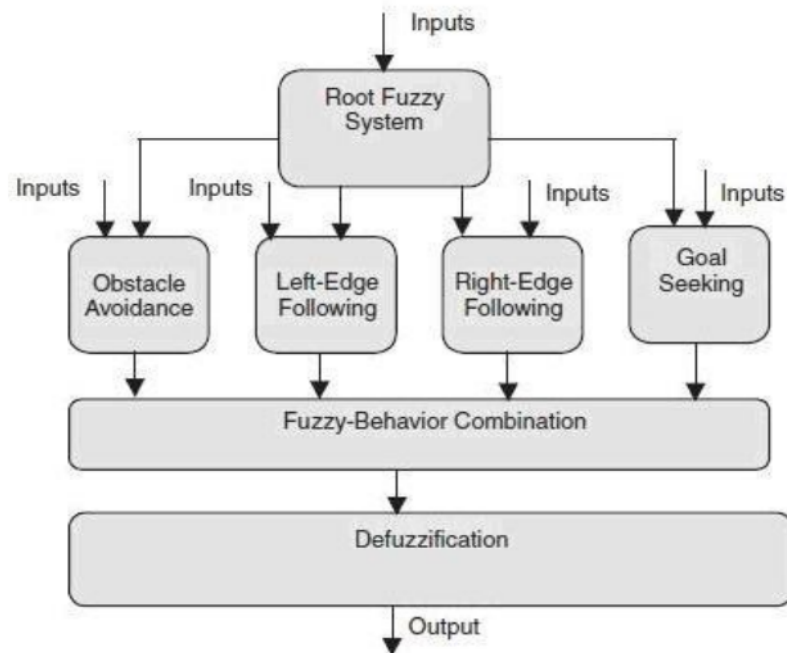
Gambar 1.4. Sistem Koordinasi Perilaku
