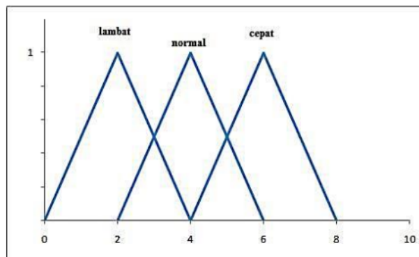
Gambar 5.2. Fungsi Keanggotaan Dari Kecepatan
