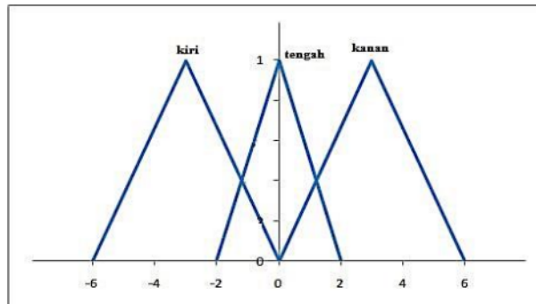
Gambar 5.3. Fungsi Keanggotaan Dari Perubahan Sudut
