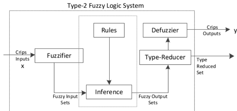
Gambar 3.5. Blok Pemrosesan SLF Tipe-2 (Karnik et. al., 1999)
