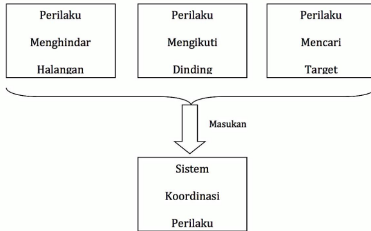
Gambar 4.14. Skema Sistem Koordinasi Perilaku
