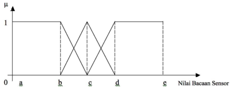
Gambar 4.16 Fungsi Keanggotaan Hirarki
