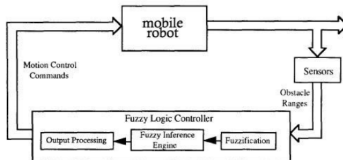
Gambar 1.3. Arsitektur SLF Pada Robot Bergerak Otonom
