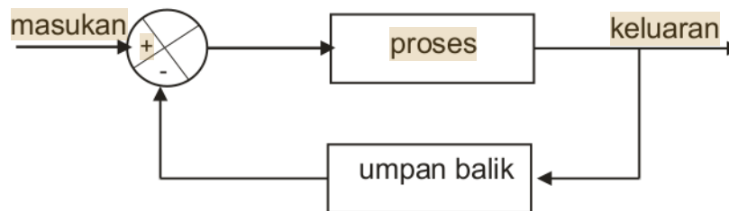
Gambar 1.2. Blok Diagram Sistem Kontrol Lup tertutup
