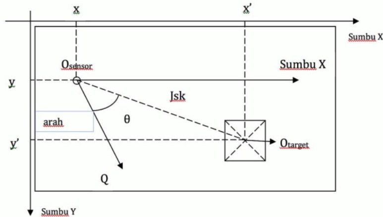
Gambar 4.10. Model Perhitungan jarak
