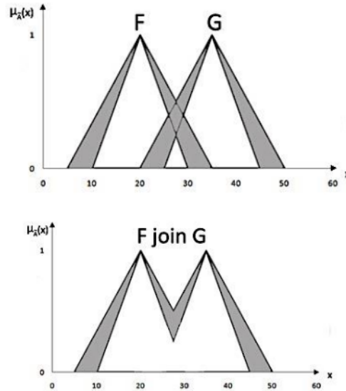
Gambar 3.9 Operasi Join Pada Himpunan Fuzzy Interval Tipe-2 (Karnik & Mendel, 2009)
