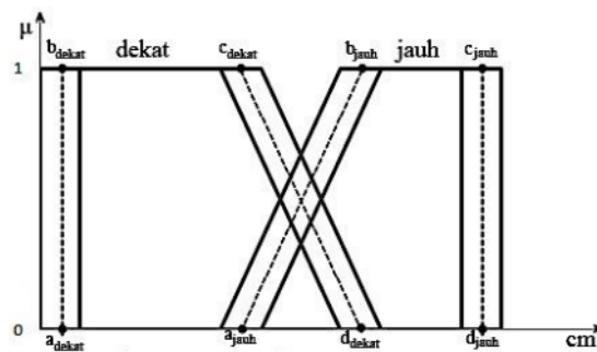
Gambar 5.6. Antecedent dari SLF penghindar halangan
