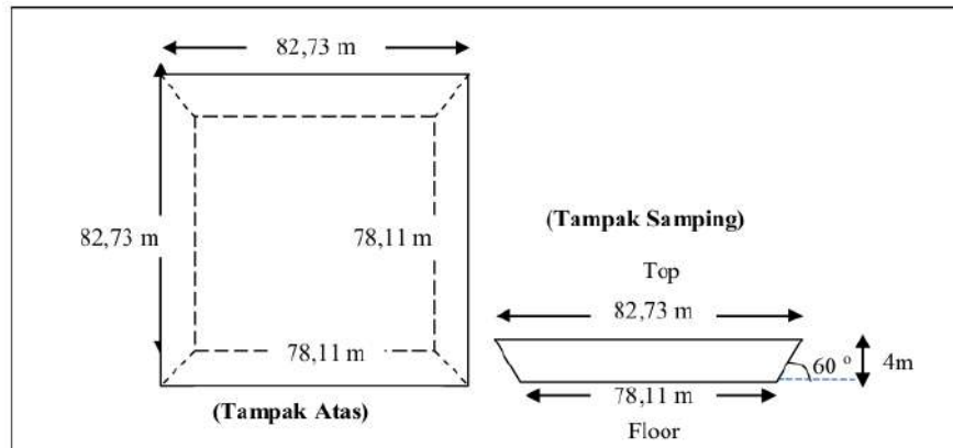
Gambar 6. Dimensi Sump Rencana PT Bumi Merapi Energi
