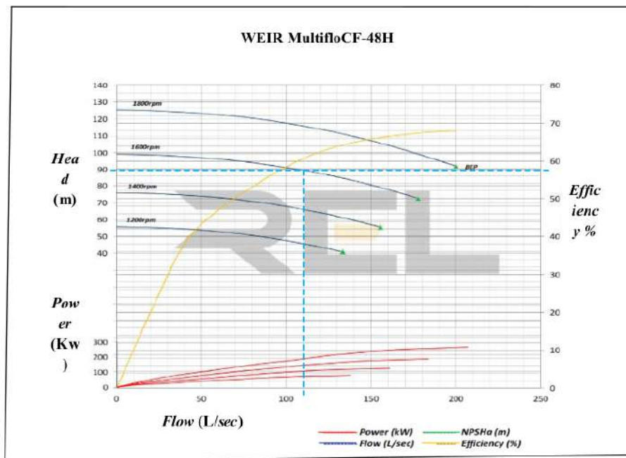
Gambar 7. Kurva Karakteristik Pompa Multiflo CF-48H
