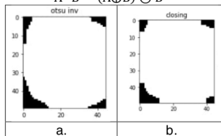
Gambar 4. (a) Hasil segmentasi dengan metode Otsu Thresholding (b) Hasil operasi morfologi dengan metode morfologi closing
