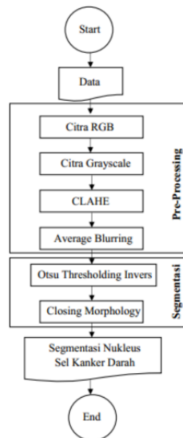
Gambar 1. Diagram alir program segmentasi menggunakan metode Thresholding
