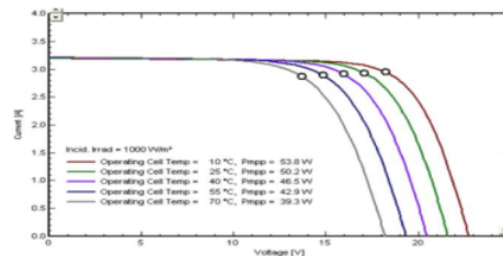
Gambar 2. Karakteristik arus (I) dan tegangan (V) modul PV (Sarhan et al., 2006)
