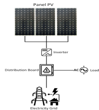
Gambar 6. Skema PLTS On-Grid
