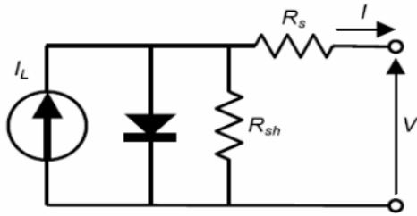
Gambar 3. Model dioda tunggal untuk rangkaian ekuivalen modul PV (Stuart R et al., 2013).
