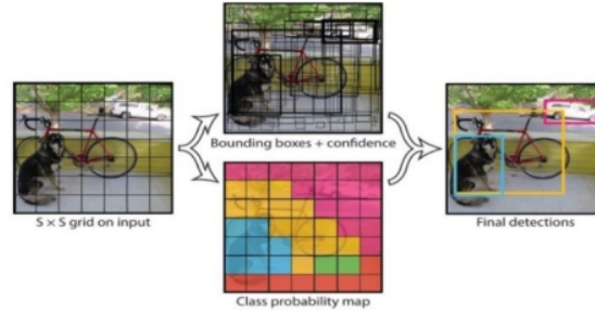
Fig. 2. YOLO Model [12]
