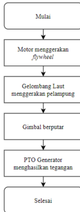
Gambar 1. Diagram Alir Kerja Sistem
