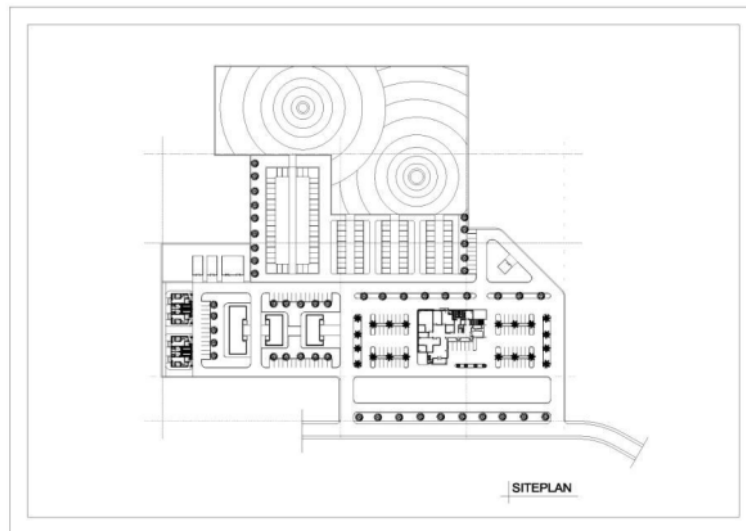
Gambar 6. Rencana Site Development Pusat Pengembangan Kerbau Pampangan Di Sumatera Selatan.
