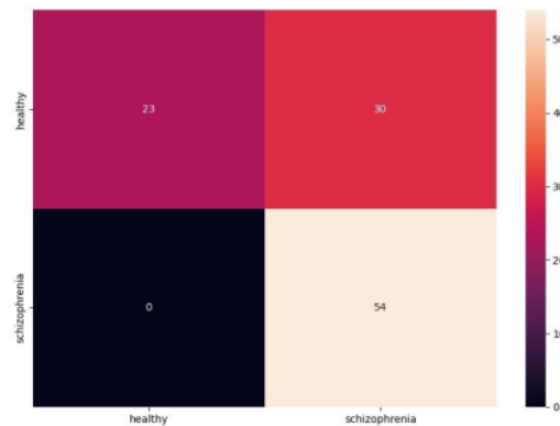
Gambar 5. Confusion Matrix Model CNN-GRU Pertama
