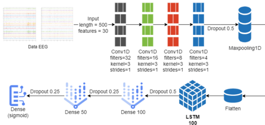
Gambar 1. Model arsitektur CNN-LSTM yang diusulkan.
