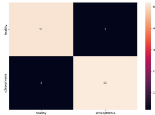
Gambar 6. Confusion Matrix Model CNN-GRU Kedua
