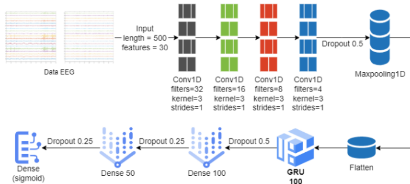
Gambar 2. Contoh Arsitektur CNN-GRU
