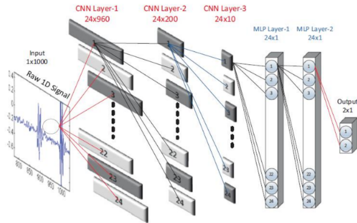
Gambar 2. Contoh arsitektur 1D CNN [14].
