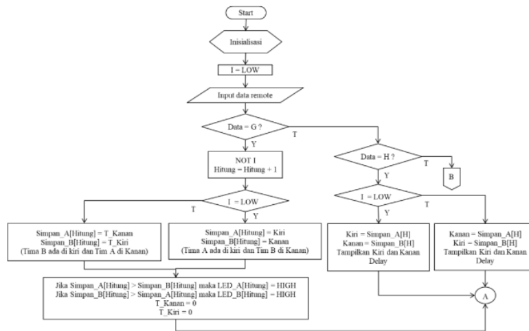
Gambar 2. Flowchart sistem keseluruhan
