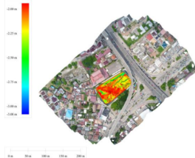
1 Gambar 11. Kedalaman yang Terukur di Semua Permukaan Kolam Retensi Simpang Pold
