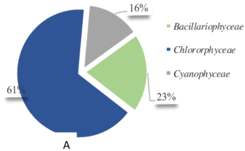
Gambar 2. Komposisi Fitoplankton di Perairan Sungai Musi Bagian Hilir. (A). Komposisi Kelas; (B). Komposisi Genus)
