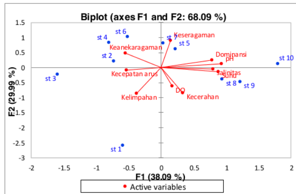
Gambar 3. Analisis Komponen Utama Sebaran Genus Fitoplankton
