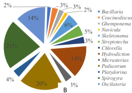
Gambar 2. Komposisi Fitoplankton di Perairan Sungai Musi Bagian Hilir. (A). Komposisi Kelas; (B). Komposisi Genus)
