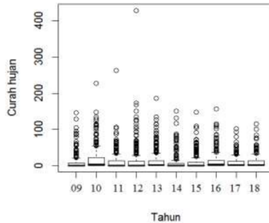
Gambar 2 Sebaran intensitas curah hujan
