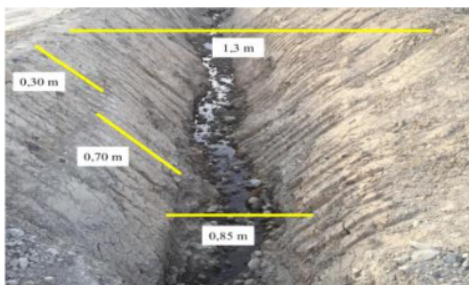
Gambar 3. Realisasi bentuk dan dimensi saluran drainase
