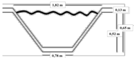
Gambar 2. Rencana bentuk dan saluran drainase
