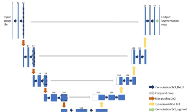
Gambar 1. Arsitektur CNN U-Net
